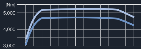
Torque V12-1400 / V12-1550
